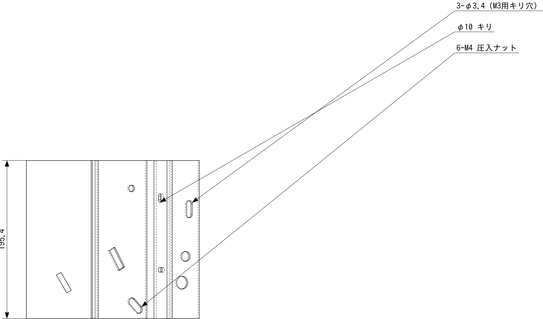
展開図（参考）
