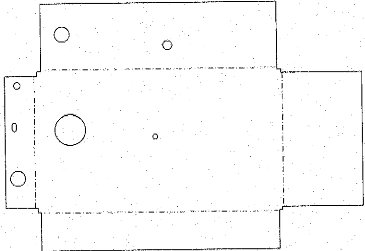
展開図 (参考)
