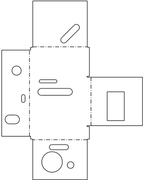
展開図（参考）
