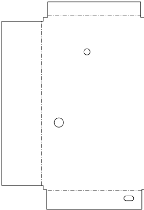
展開図（参考）
