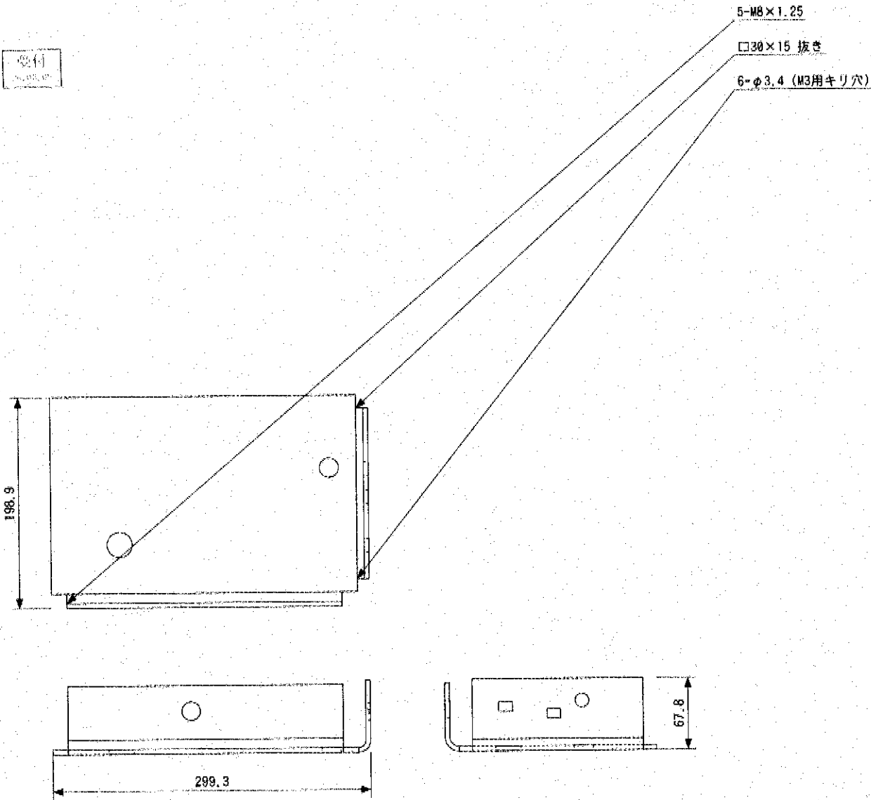
展開図 (参考)
