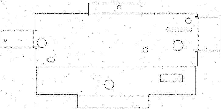
展開図 (参考)
