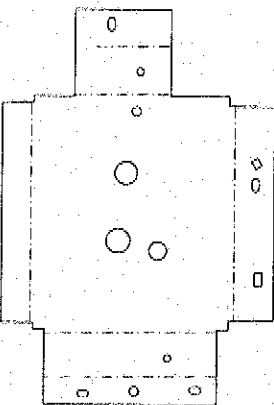
展開図 (参考)
