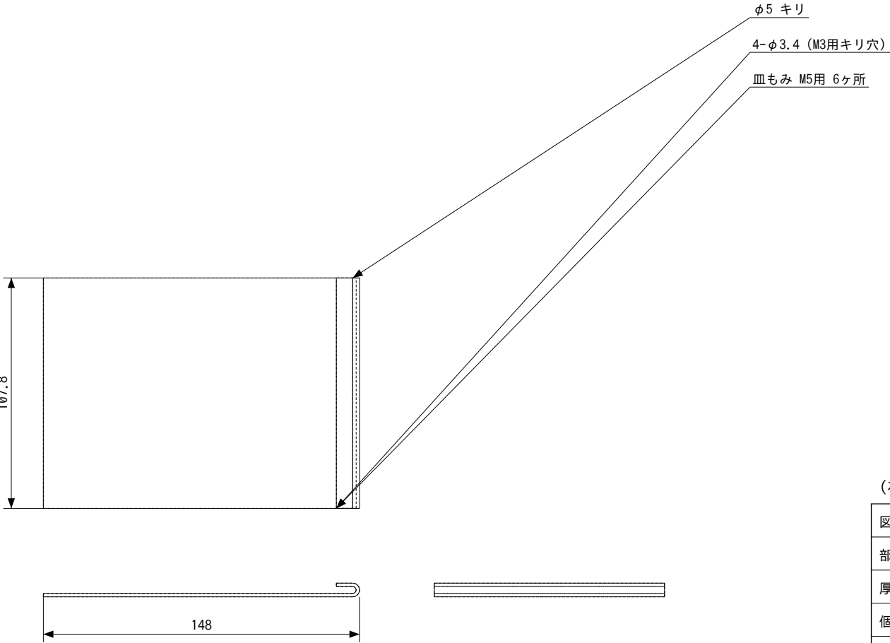
展開図（参考）
