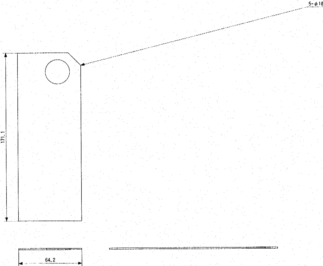
展開図（参考）
