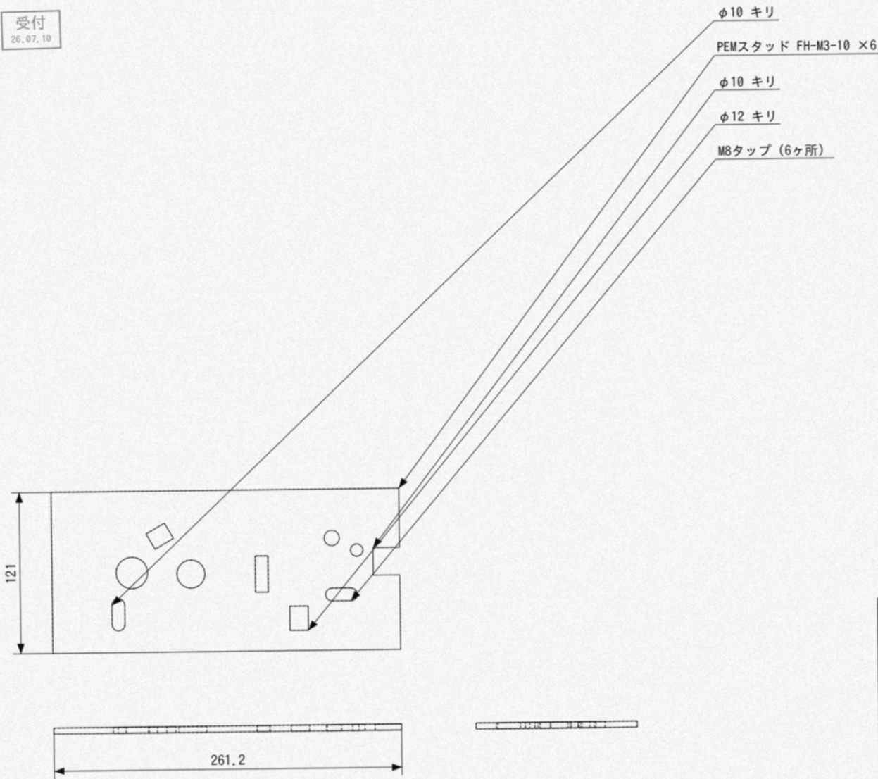
展開図 (参考)
