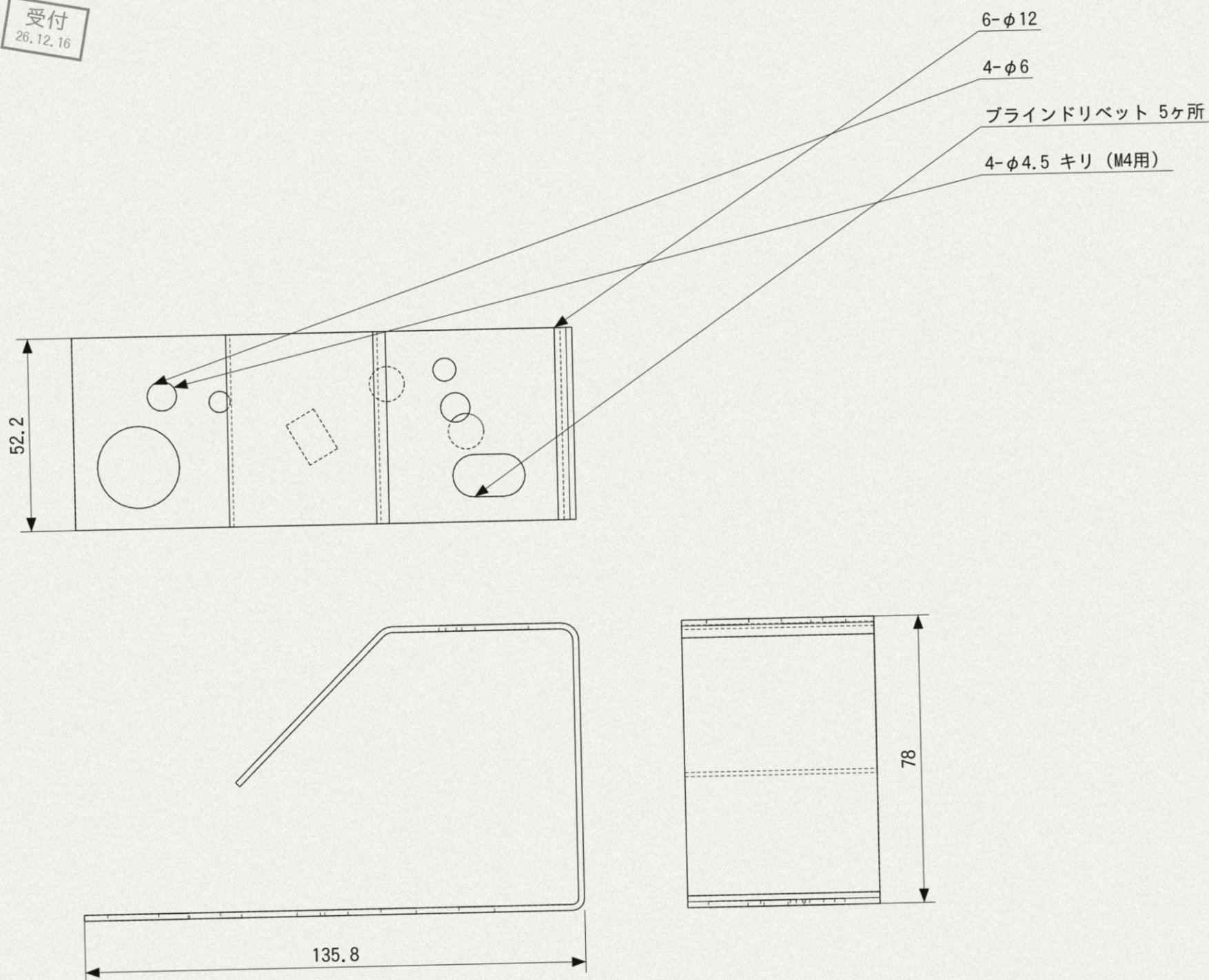
展開図（参考）
