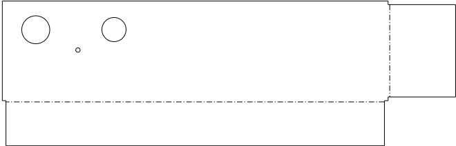
展開図（参考）
