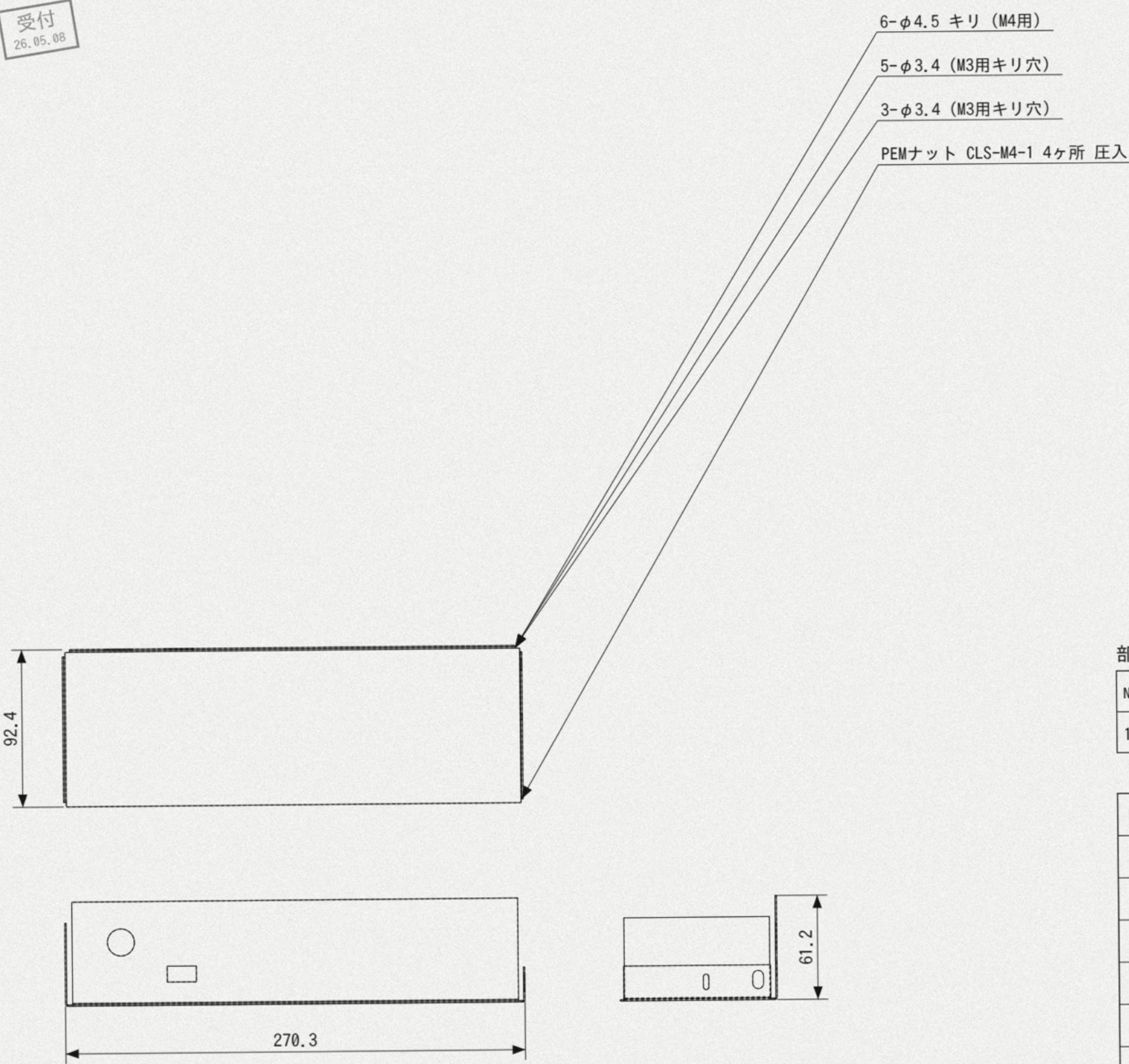
展開図 (参考)
