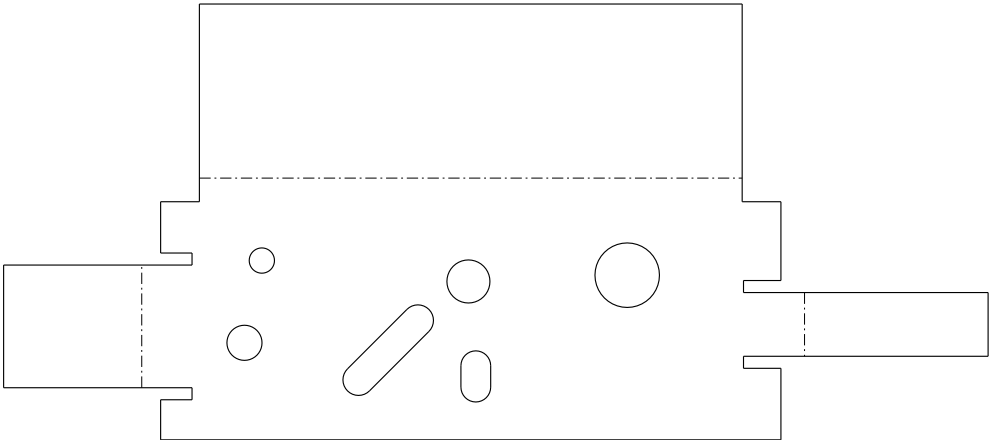
展開図（参考）
