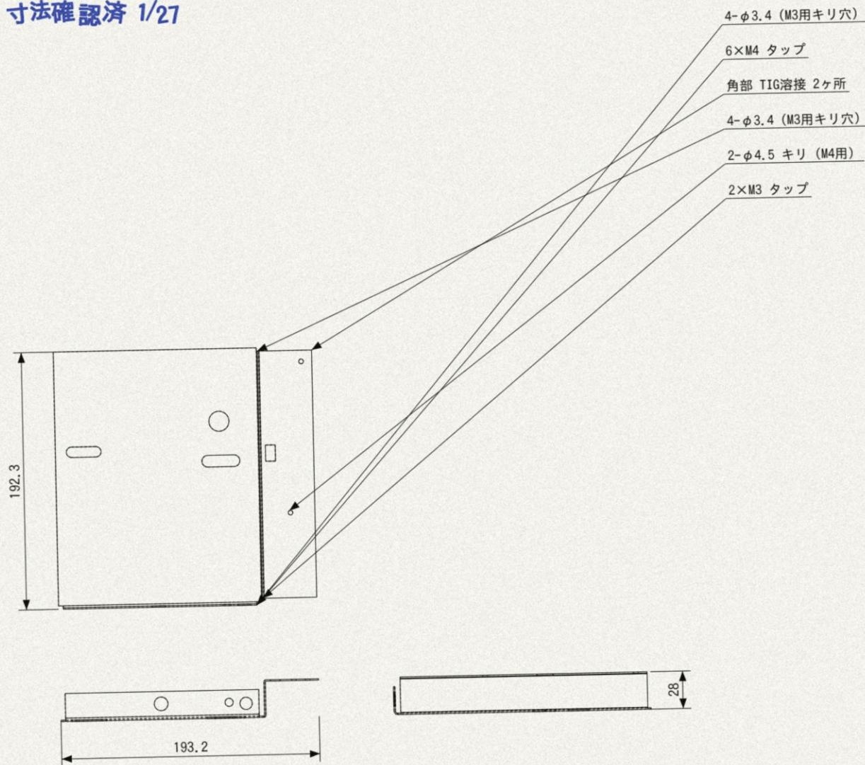
展開図 (参考)
