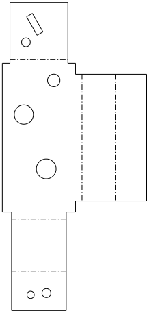
展開図 (参考)
