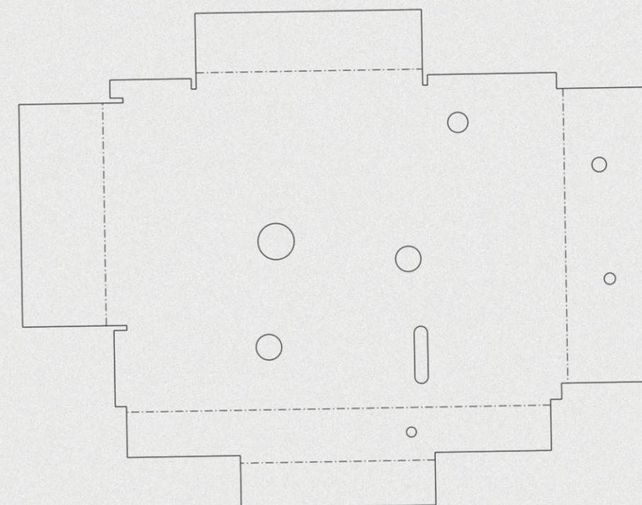
展開図 (参考)
