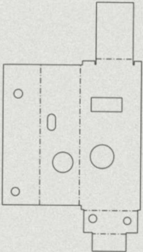
展開図（参考）
