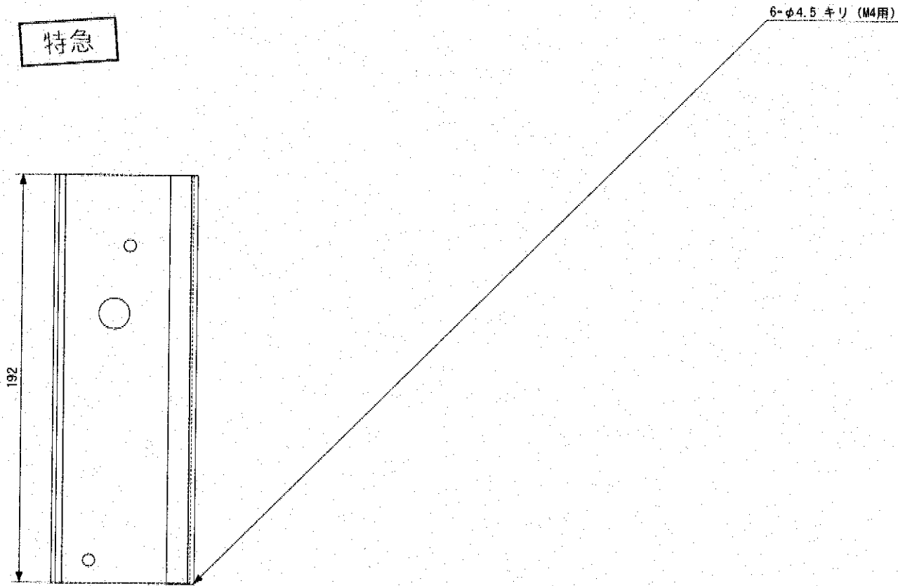
展開図 (参考)
