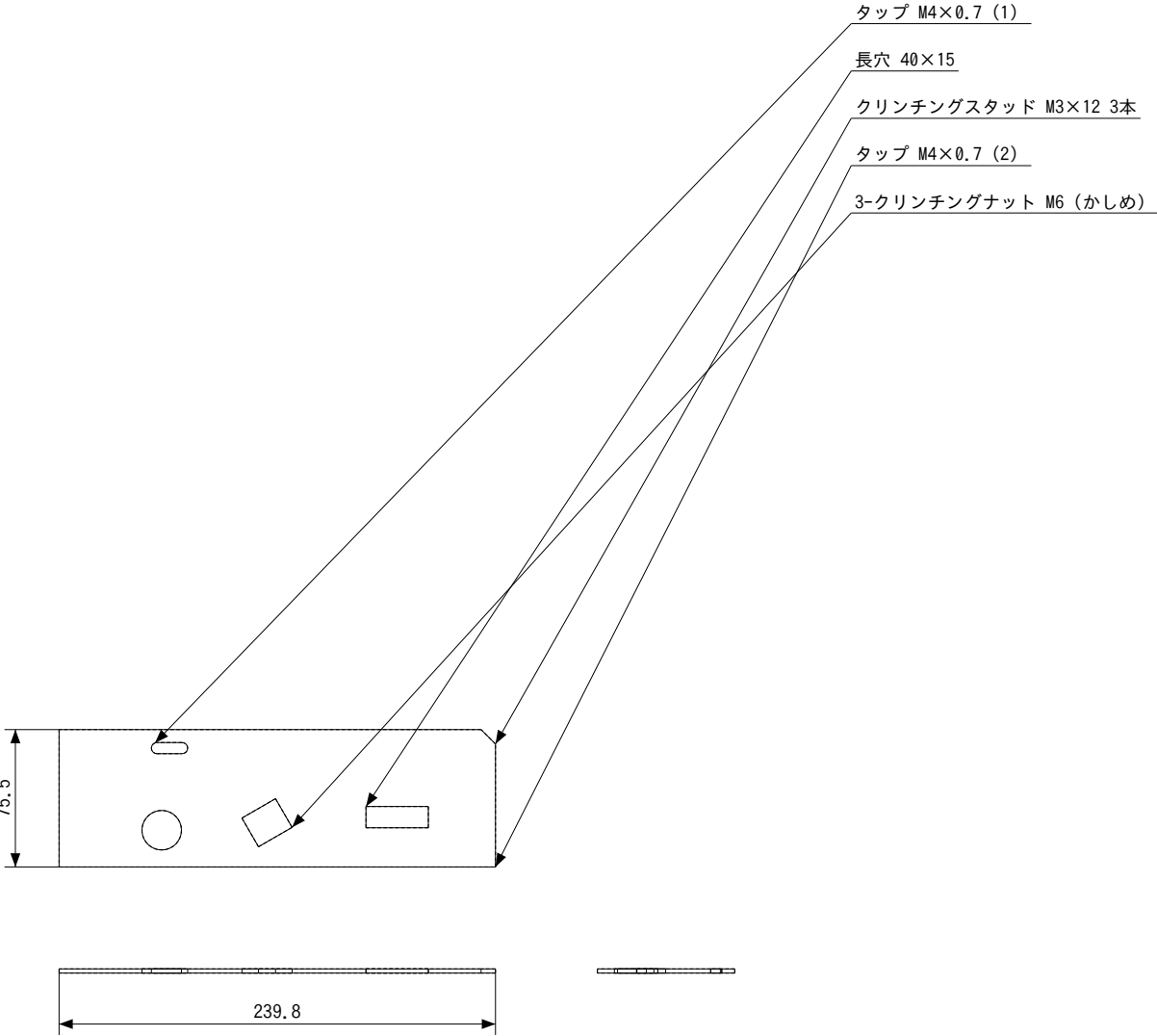
展開図（参考）
