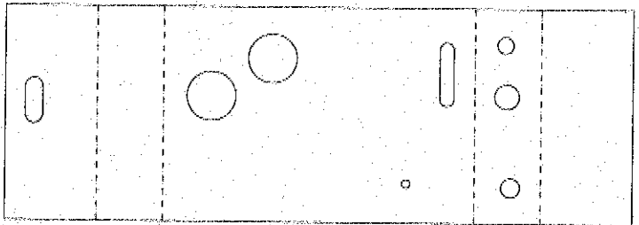
展開図 (参考)
