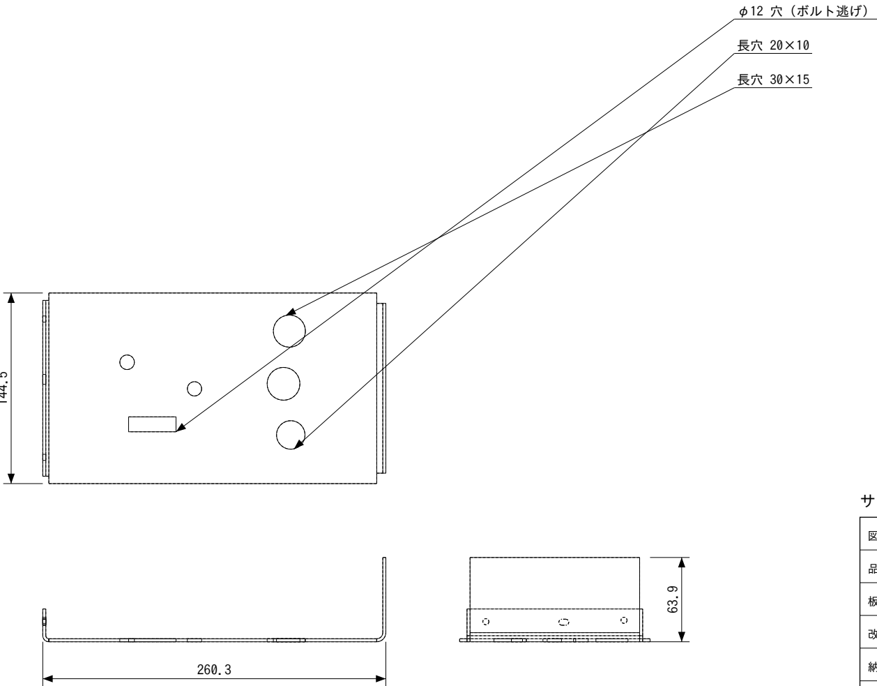
展開図 (参考)
