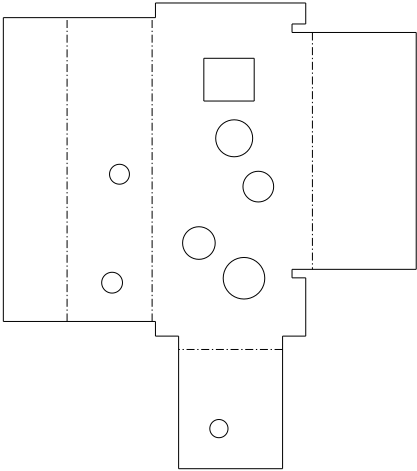
展開図 (参考)
