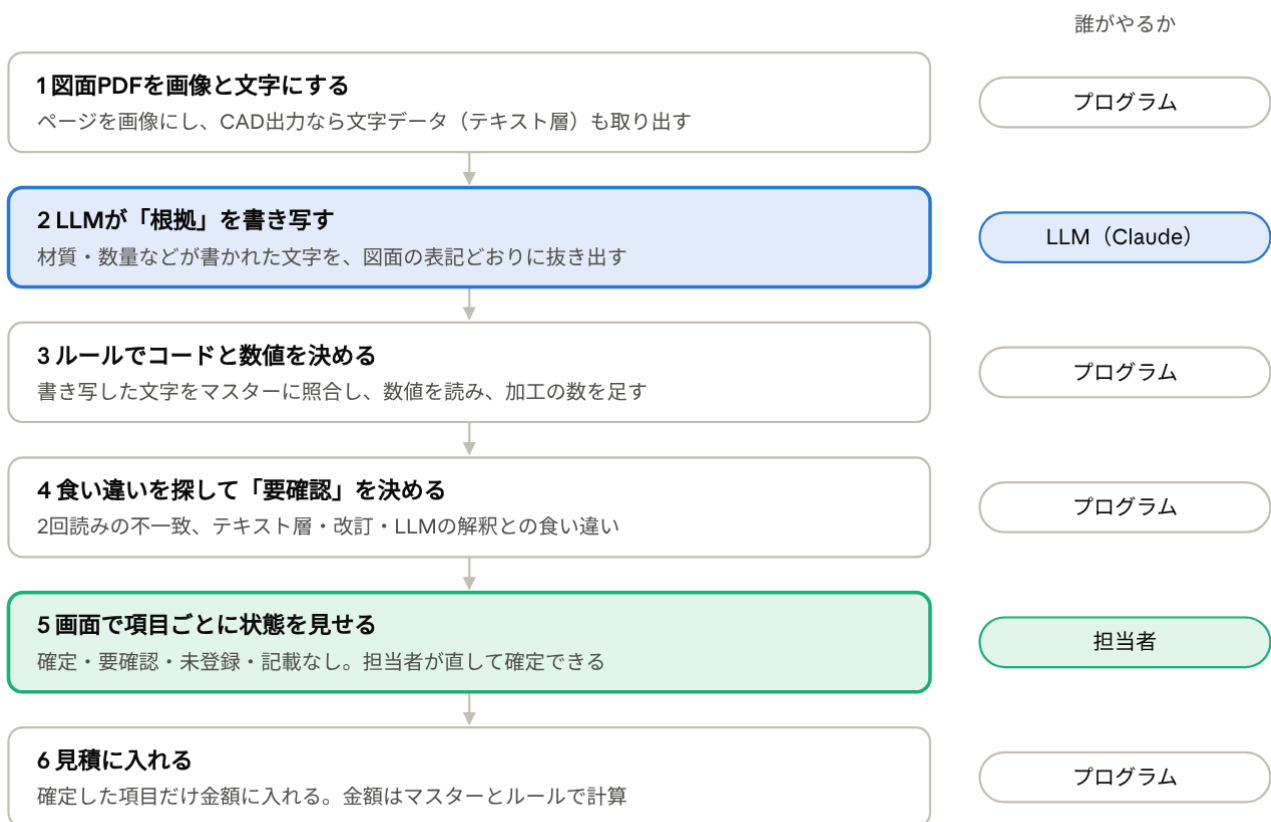
図面PDF読み取りの流れ（LLMは書き写すだけで、値を決めるのはルール）
