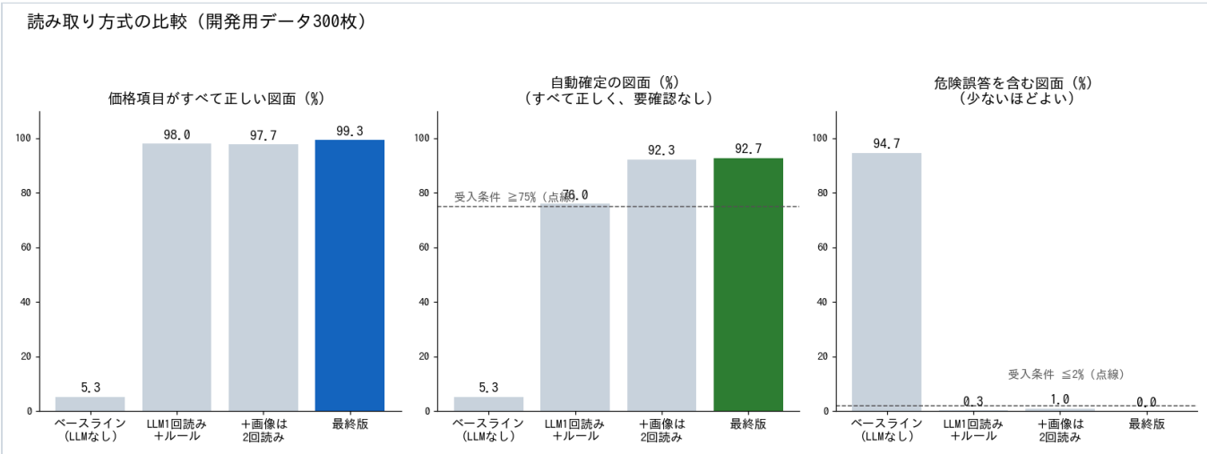
読み取り方式の比較
