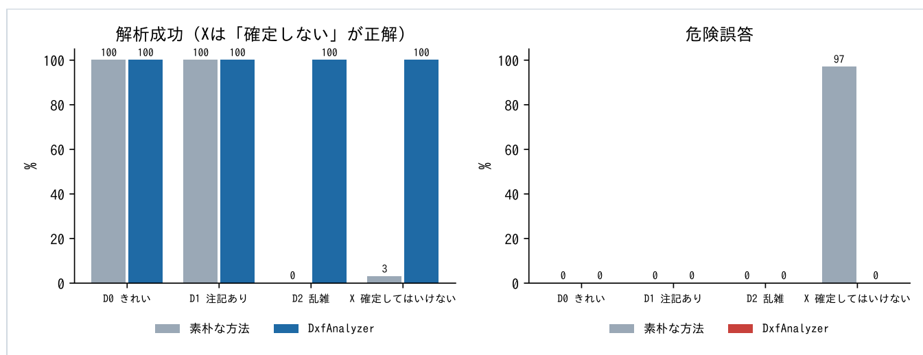
素朴な方法との比較（開発用800ファイル）
