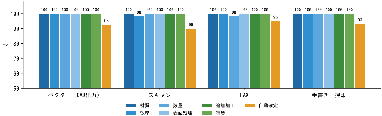
図面PDF：PDFの種類別の正解率と自動確定（開発用 300枚）
