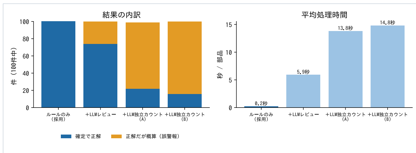
LLMを足した方式との比較
