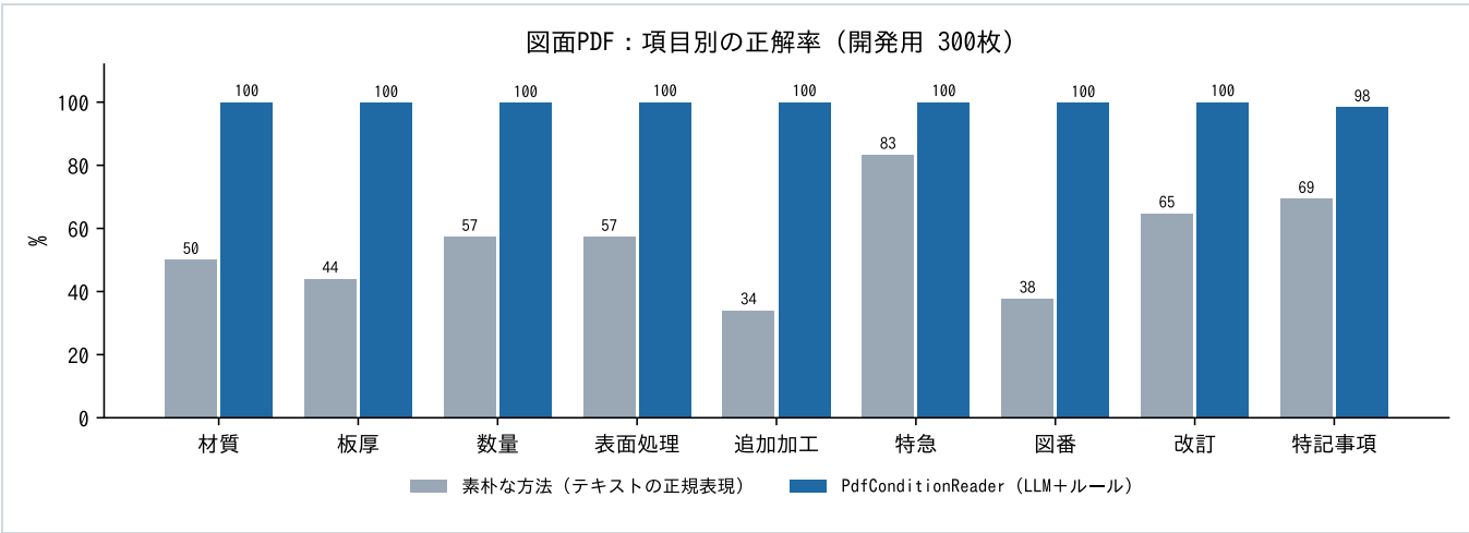
項目別の正解率：素朴な方法との比較
