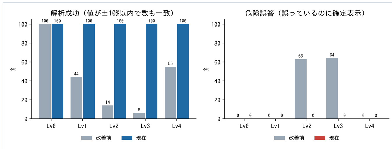
改善前と現在の比較（開発用508件）
