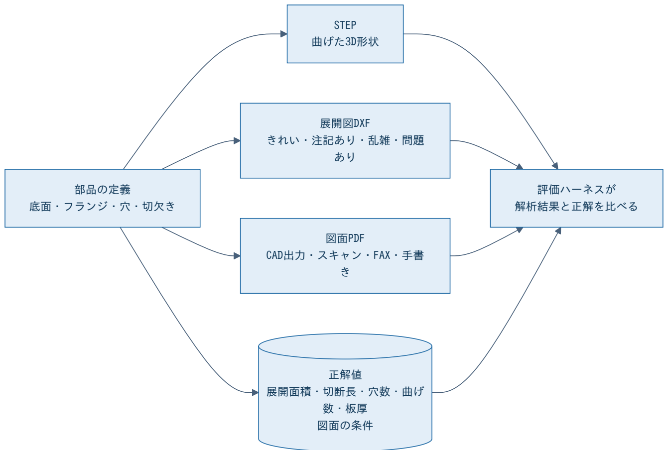
図 ゴールデンデータの作り方：正解を先に決め、描き方だけを変える
