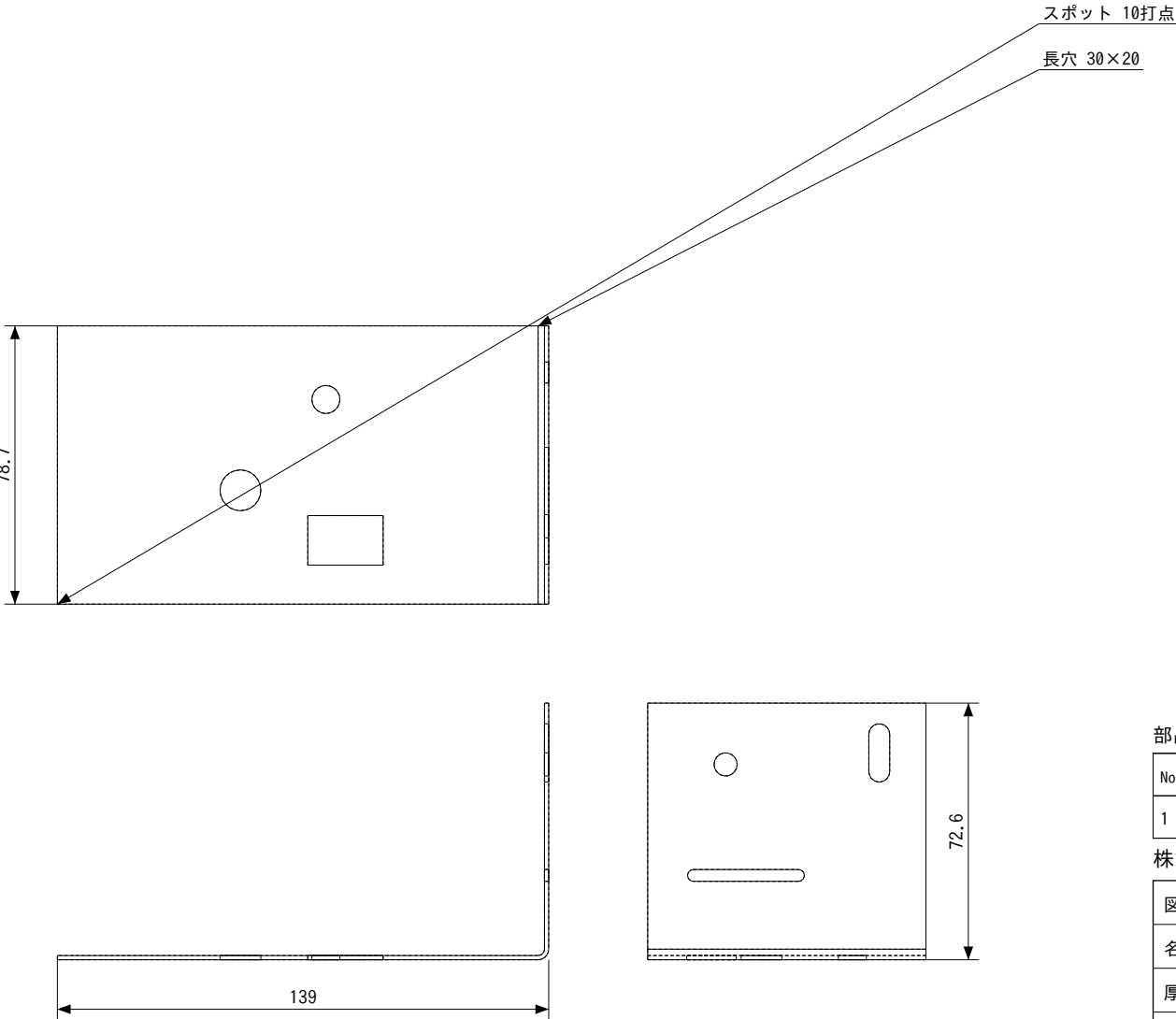
展開図（参考）
