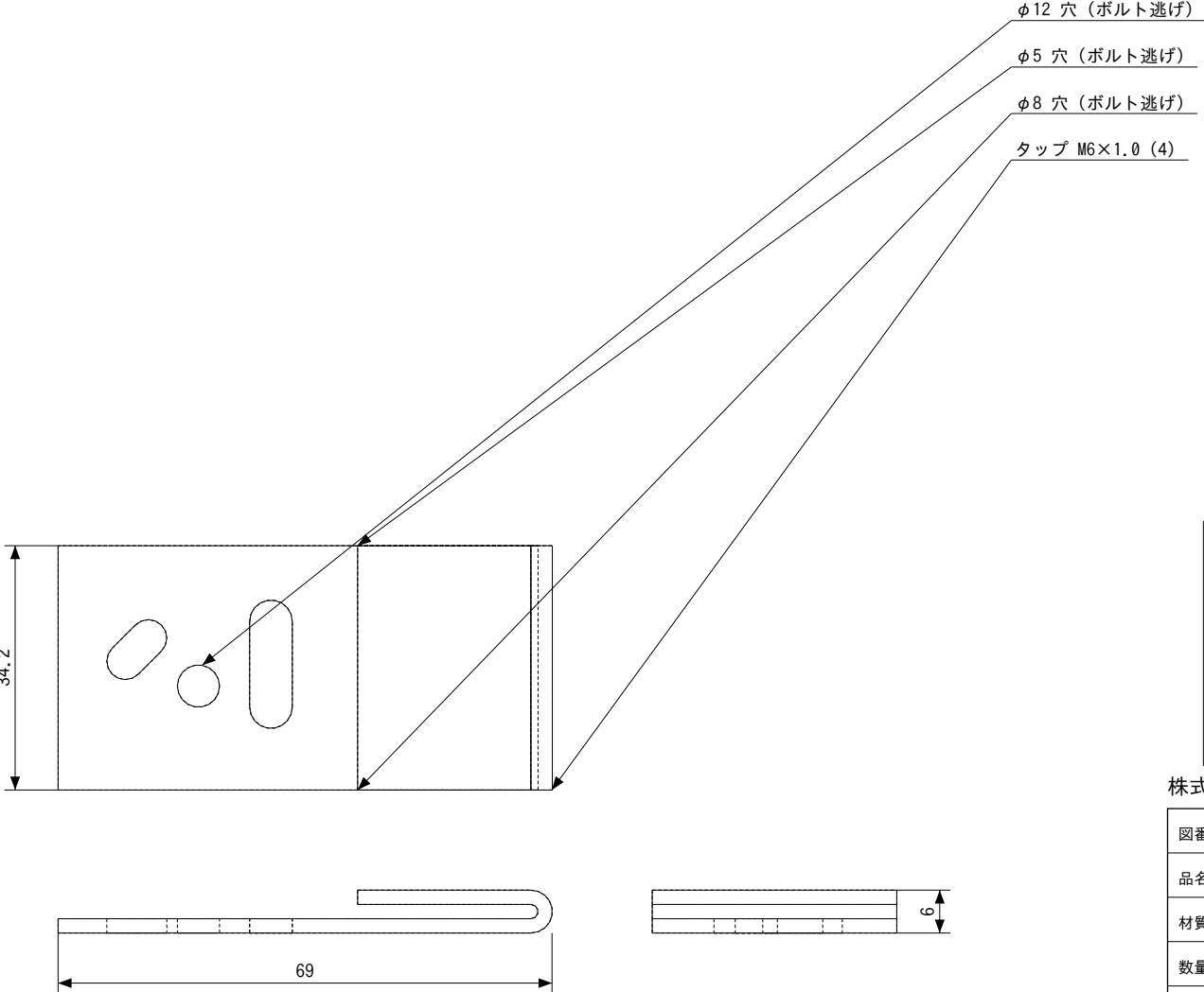
展開図 (参考)
