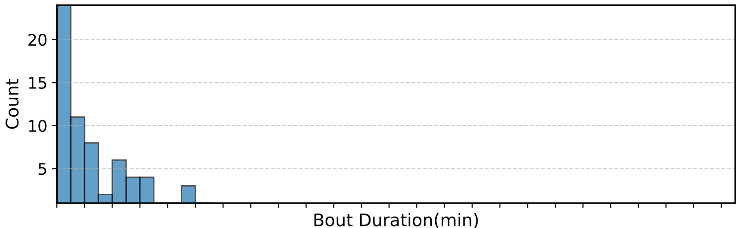
SC13(Control
