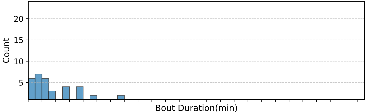
SC14(Control
