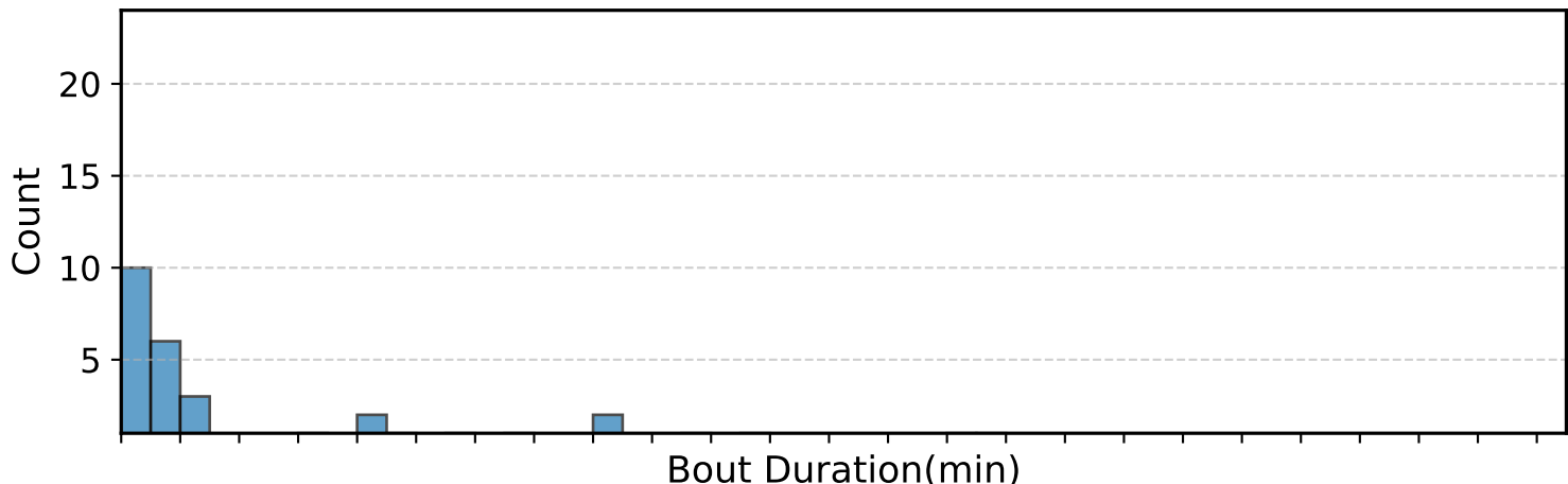
SC09(SNr-DTA)
