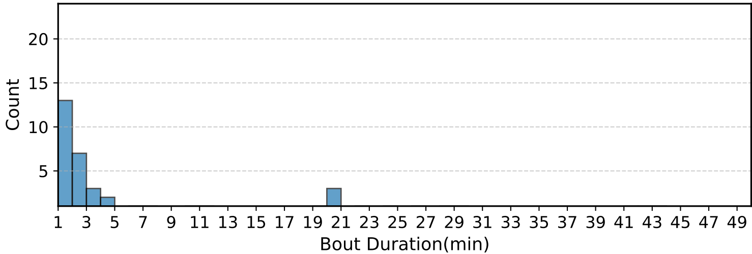
SC15(Control
