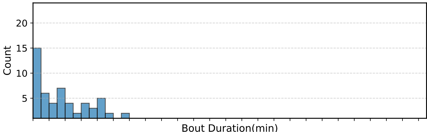
SC11(SNr-DTAY
