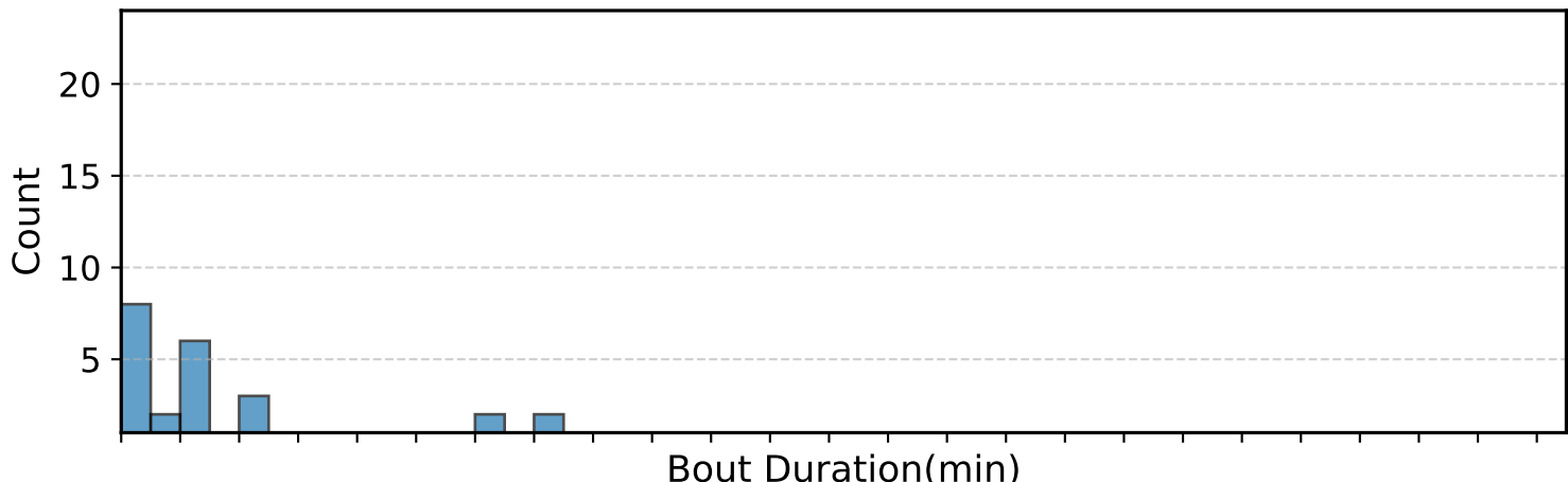
SC12(SNr-DTA)
