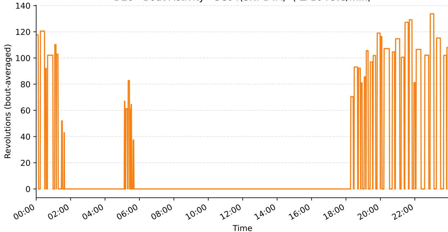
D20 - Bout Activity - SC04(SNr-DTA) ( \geq 10 revs/min)
