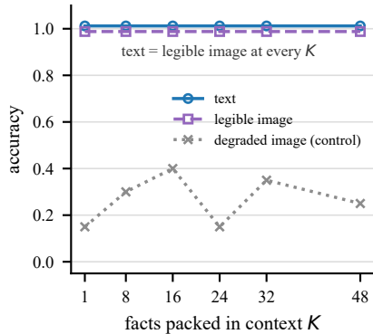
Frontier retrieval: Gemini 3.1 Pro
