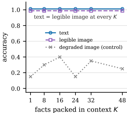
E8 retrieval: Gemini 3.1 Pro
