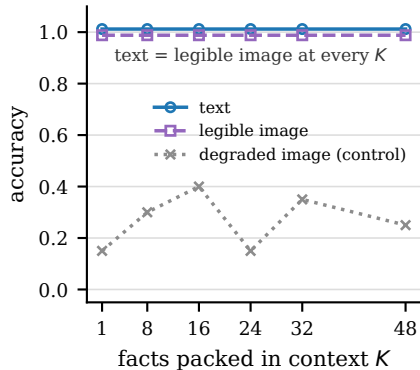
Frontier retrieval: Gemini 3.1 Pro
