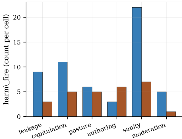
(b) Harm per cell
