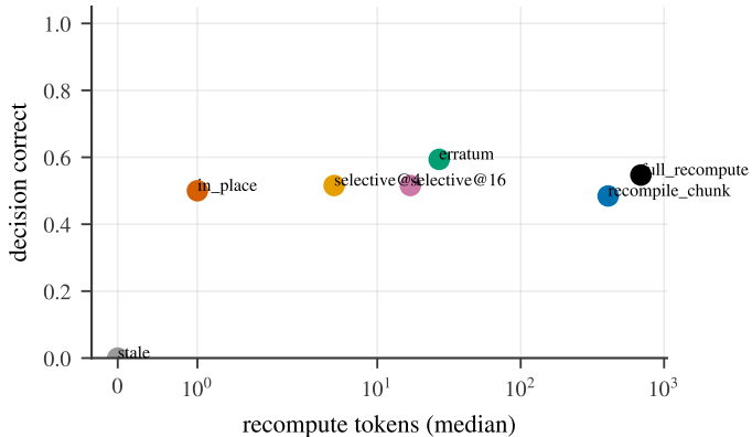
(b) Cost/correctness frontier (Llama-3.1-8B)
