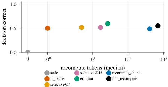
(b) Cost/correctness frontier (Llama-3.1-8B)
