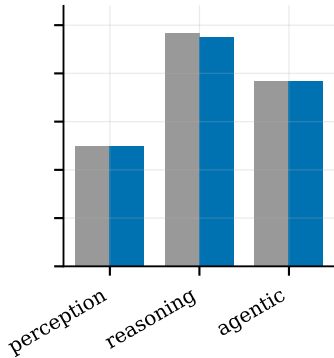
Qwen3-VL-8B
