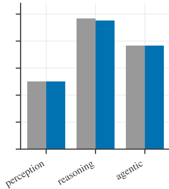
Qwen3-VL-8B
