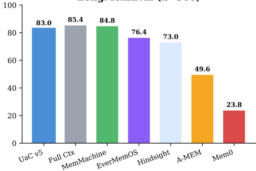
LongMemEval (n=500)
