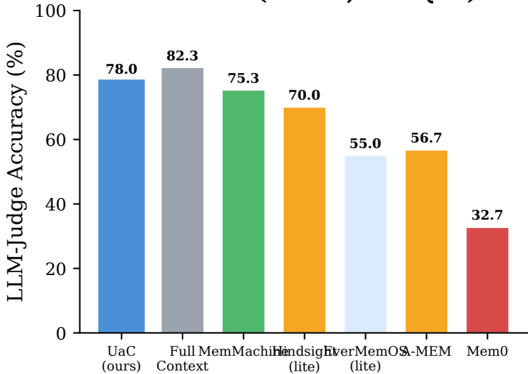
LOCOMO (5 conv, 300 QAs)
