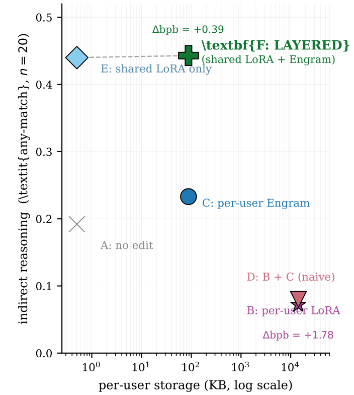
(d) Pareto on Mini-Engram-d20 (same base, six substrate combos)
