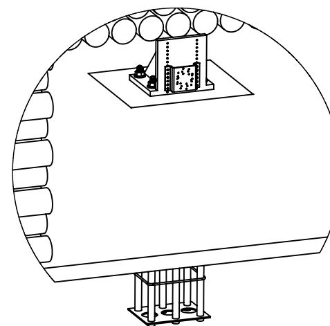
DETALHE A ESCALA 1 : 20
