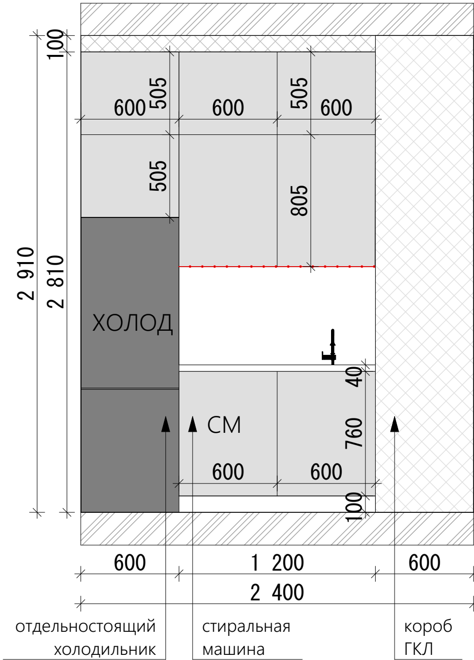
Развертка кухонной мебели
