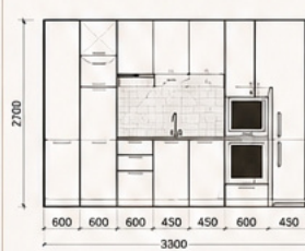
РАЗВЕРТКА КУХОННОЙ МЕБЕЛИ
