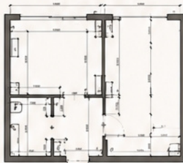
ПЛАН ДЕМОНТАЖА
