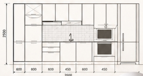
РАЗВЕРТКА КУХОННОЙ МЕБЕЛИ
