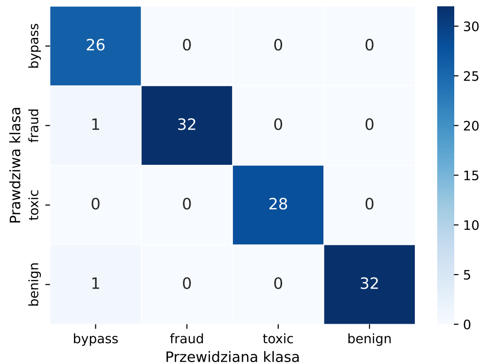
Modul C (HerBERT)
