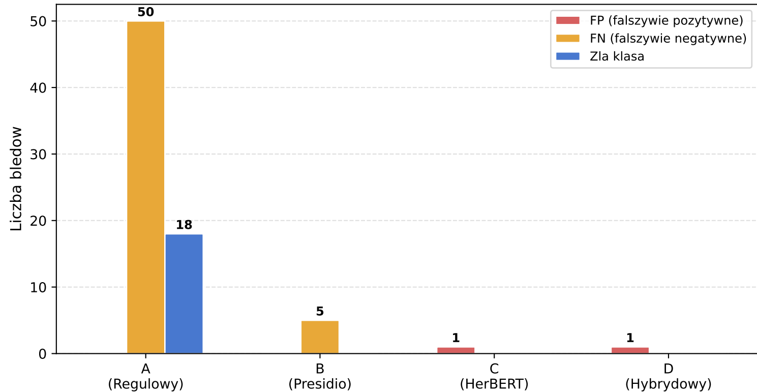
Bledy klasyfikacji (zbior testowy, n=120)
