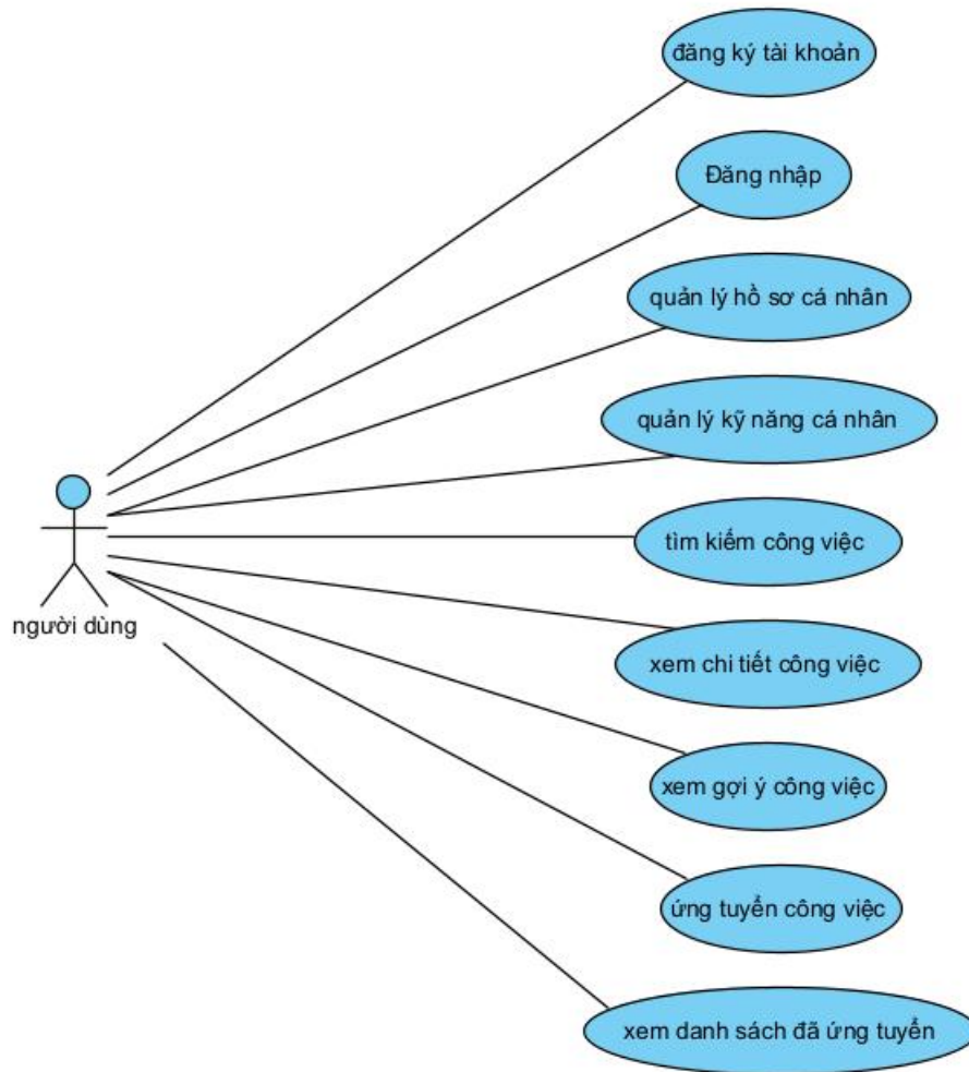
Hình 3.4 Biểu đồ Usecase tác nhân người dùng
