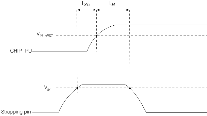
图 2: Strapping 管脚的时序参数图
