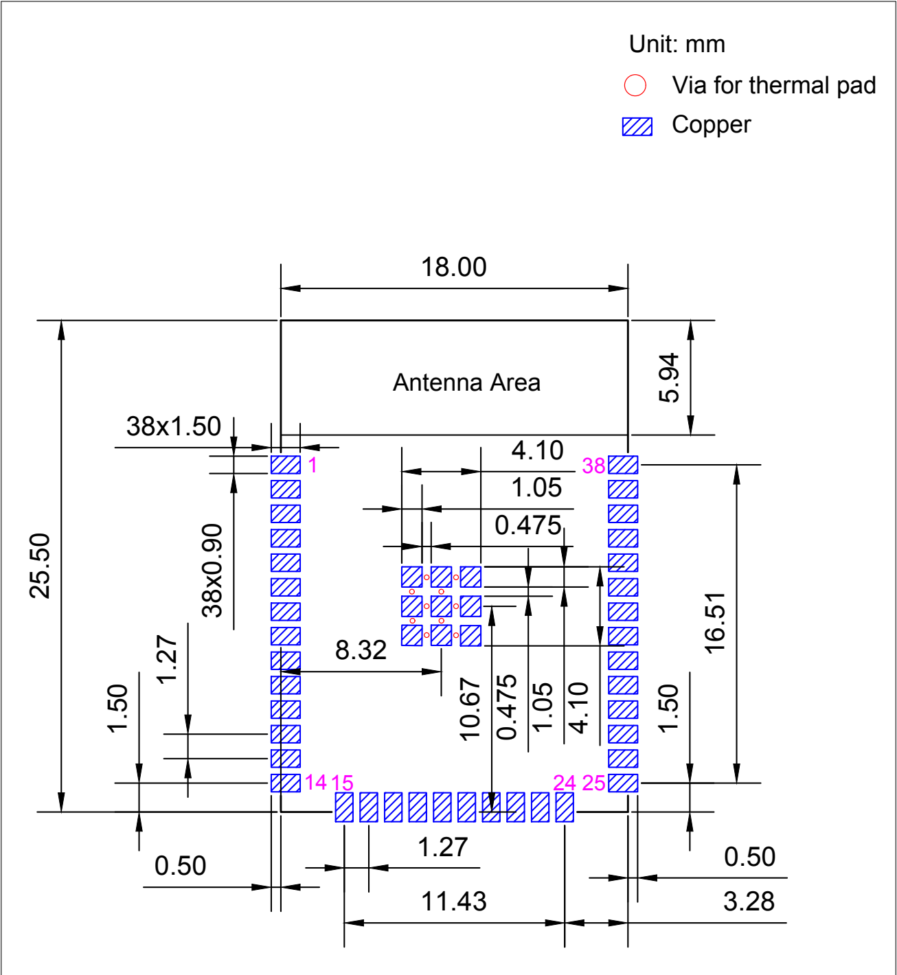
图 8: 推荐 PCB 封装图形
