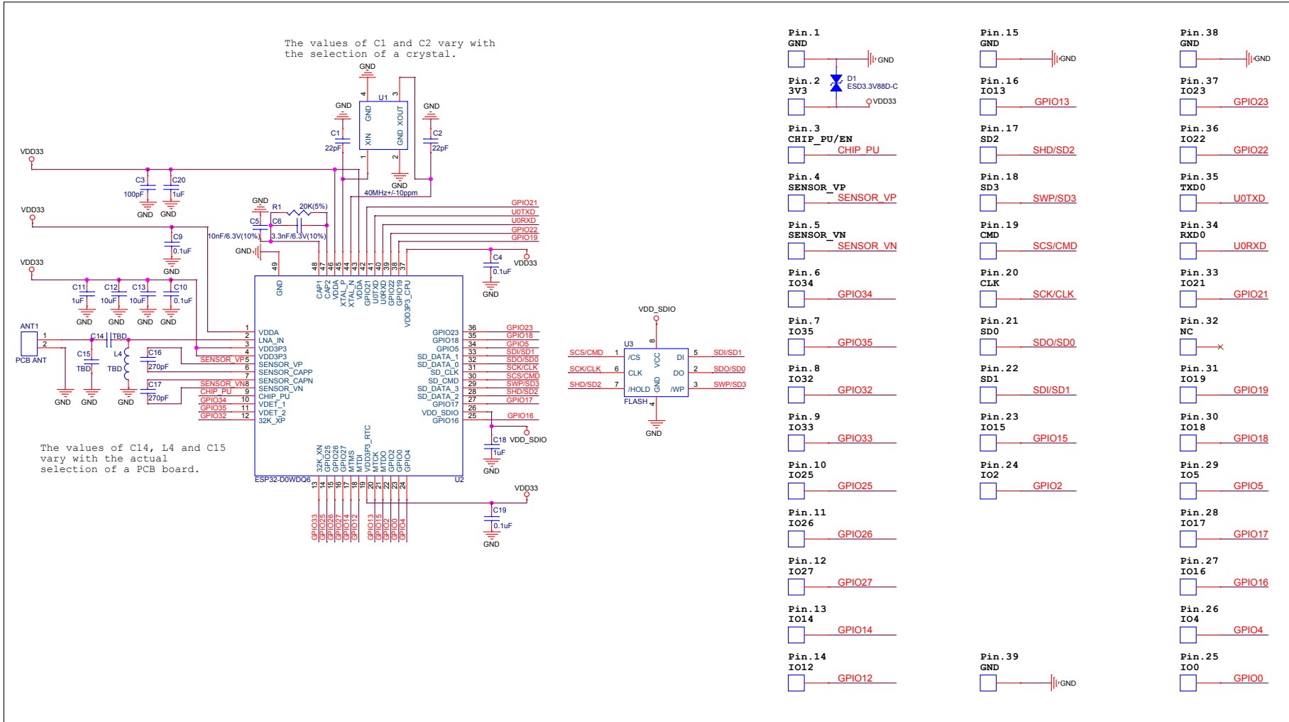
图 5: ESP32-WROOM-32 原理图
