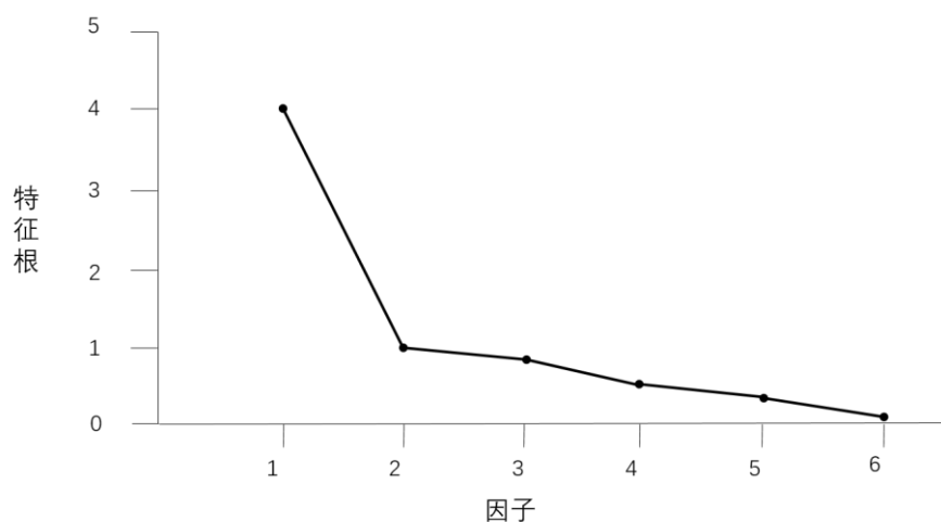
图 3-3 碎石图
