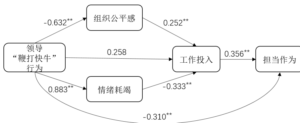
图 4-1 结构方程模型
