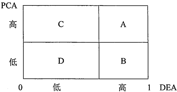
图 2.2 DEA/PCA 相结合评价方法示意图
