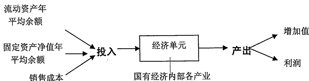
图 2.1 DEA 评价方法示意图
