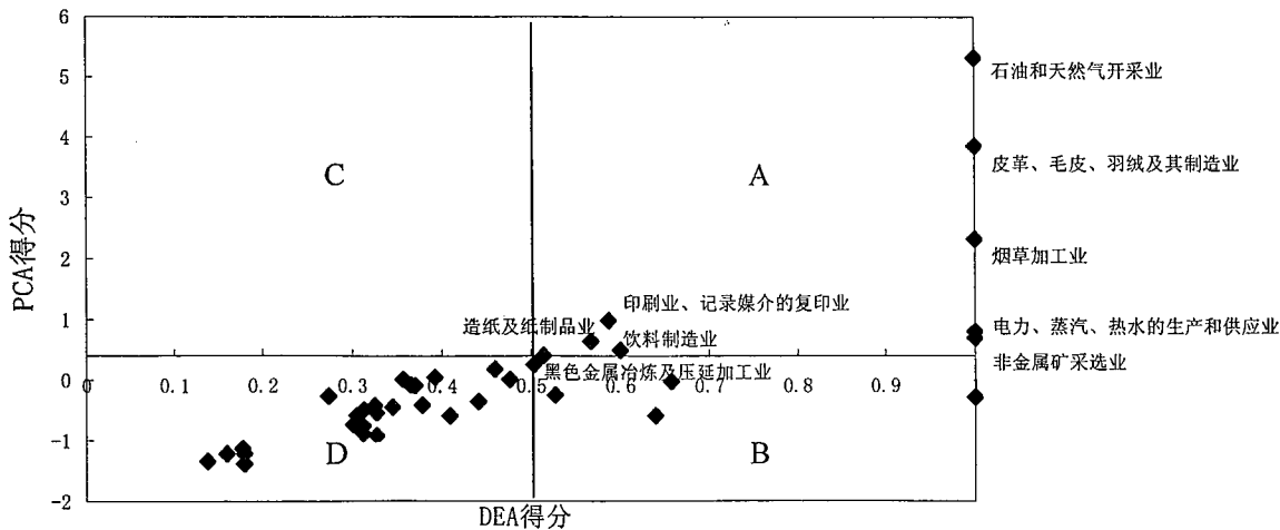
图3.4 DEA和PCA相结合分析图
